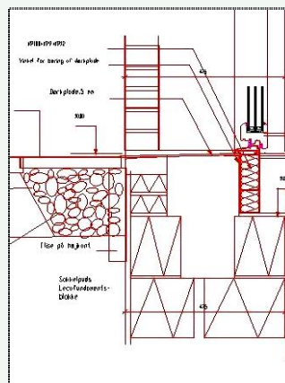
Illustr.: Suensons Tegnstue Fundamentsokkel
