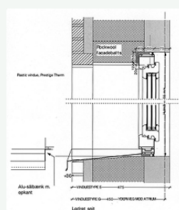
Grafik: Suensons Tegnestue Detaljer vinduesmontering
